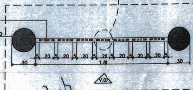
01 DETALHE GUARDA CORPO escala: 1/20
