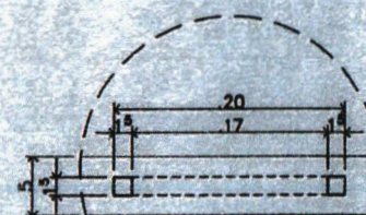
DETALHE - PLANTA PEÇA EM FERRO ESC: 1/5
