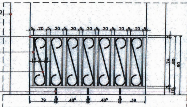
02 VISTA 03 escala: 1/20
