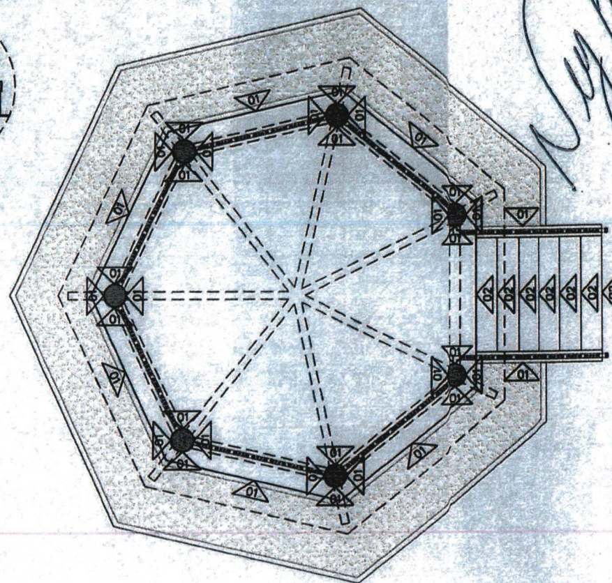
01 PLANTA DE REVESTIMENTOS-CORETO escala: 1/50
