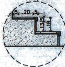
DETALHE CORTE ESCADA ESC: 1/20
