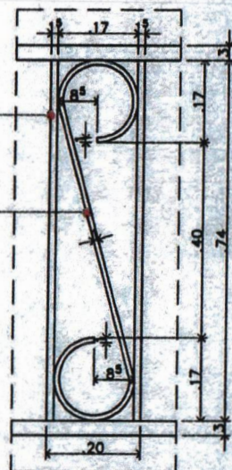
03 DETALHE - VISTA PEÇA EM FERRO escala: 1/10
