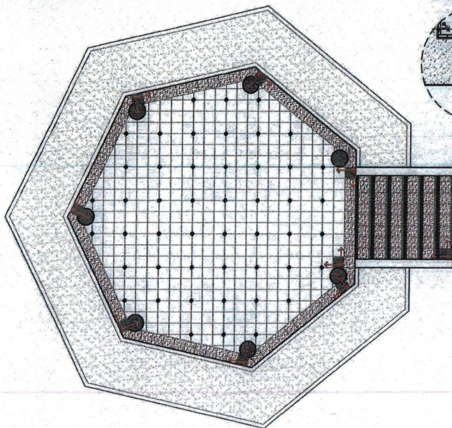
02 PLANTA DE PAGINAÇÃO DE PISOS-CORETO escala: 1/50
